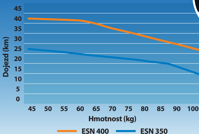
Dojezd (km) v závislosti na hmotnosti (kg)
